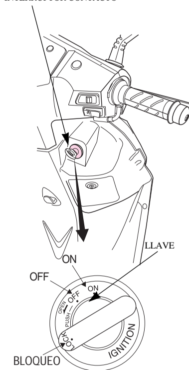
INTERRUPTOR CONTACTO
