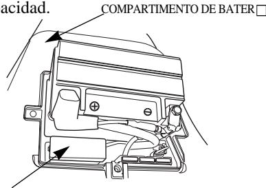
PORTAFUSIBLES
