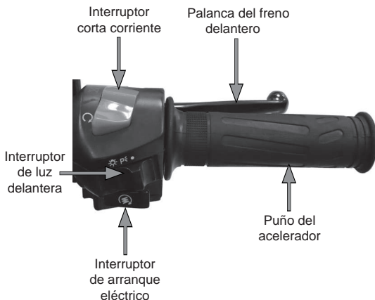
Imagen 5. Mando derecho
