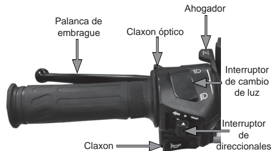
imagen 8. Mando izquierdo
